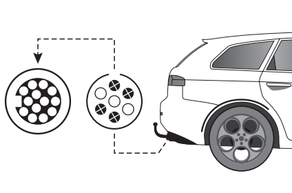
Thule Adapter 9906 – Převádí elektrickou zásuvku automobilu s 7 pólů na zásuvku se 13 pólů.
